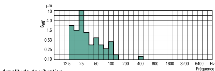
Amplitude de vibration
