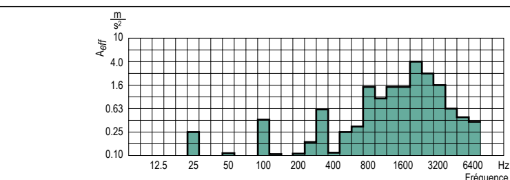
Accélération de vibration
