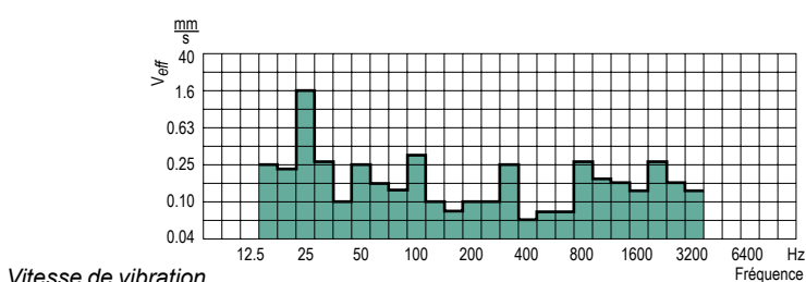
Vitesse de vibration
